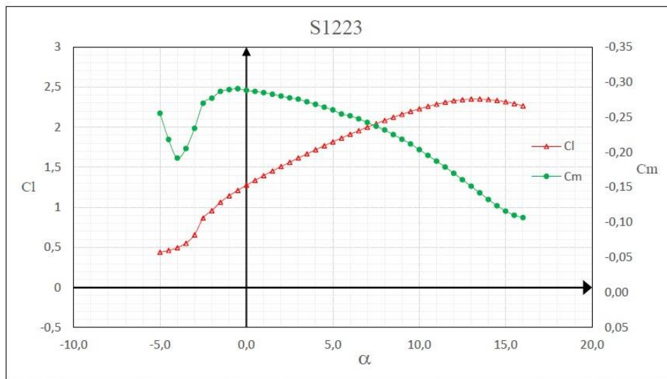
Figura 12: C_l x C_m do perfil S1223.
