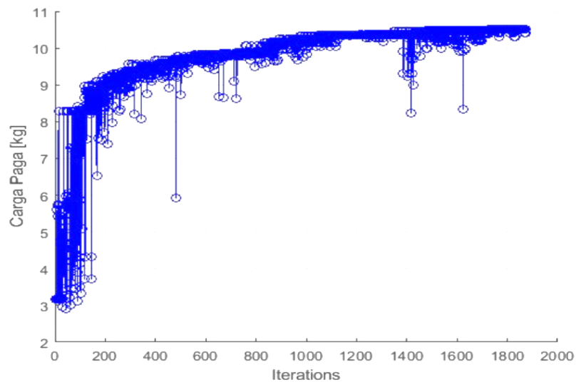
Figura 17: Curva de otimização para o projeto de 2020.
