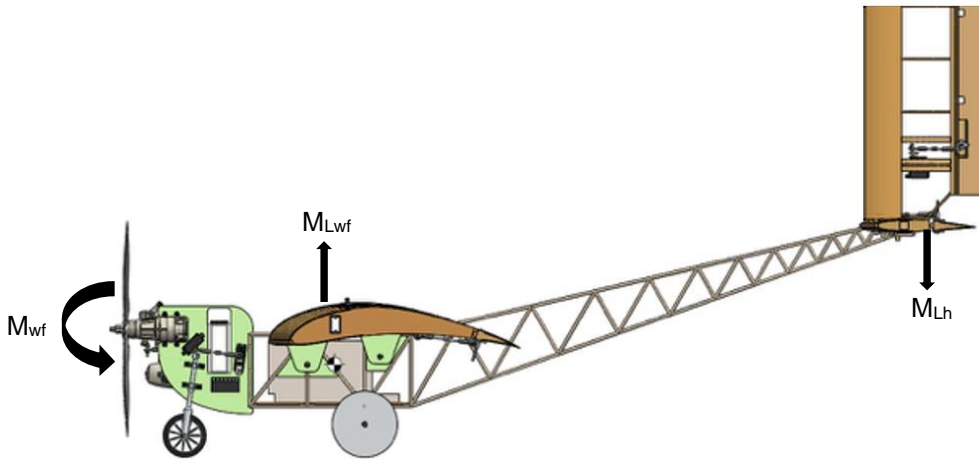
Figura 6: Momentos atuantes no eixo longitudinal da aeronave.
