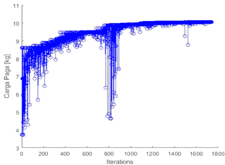
Figura 14: Gráfico de evolução do algoritmo até a convergência.
