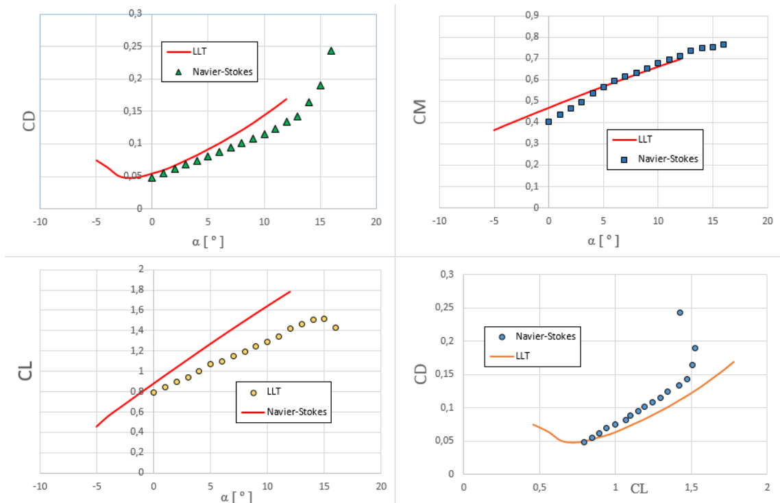
Figura 9: Comparativo do método LLT com a solução numérica ANSYS® CFX.
