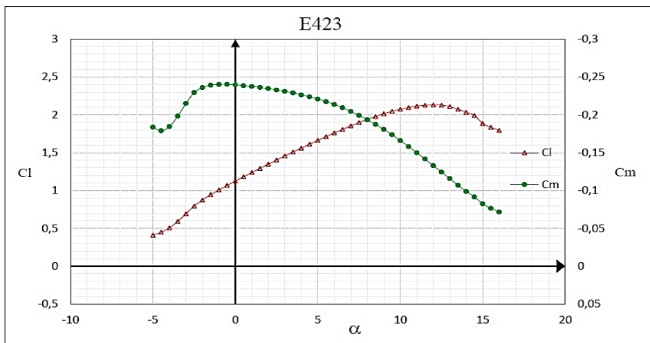
Figura 11: C_l x C_m do perfil E423.
