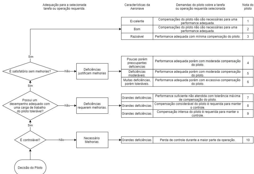
Figura 15: Escala Cooper Harper para testes de controlabilidade.
