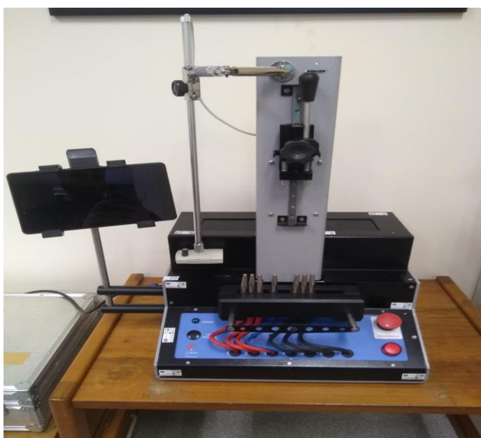
Figura 10 – Bancada Trifásica M-3.
