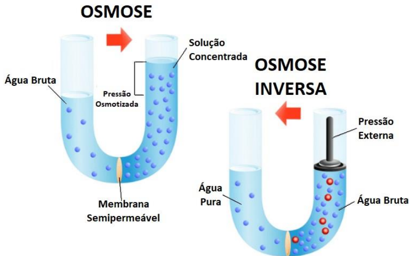
Figura 1: Representação do funcionamento da técnica de osmose
