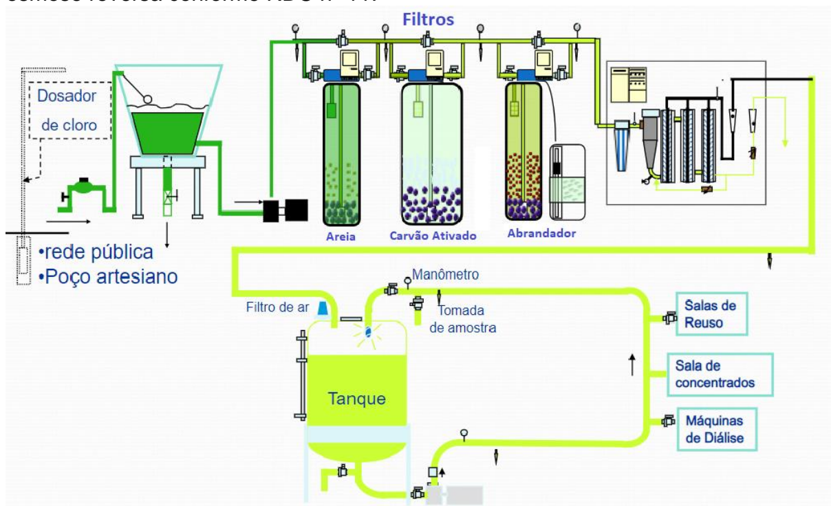
Figura 2: Sistema de pré-tratamento da água antes da passagem pela membrana de osmose reversa conforme RDC nº 11.
