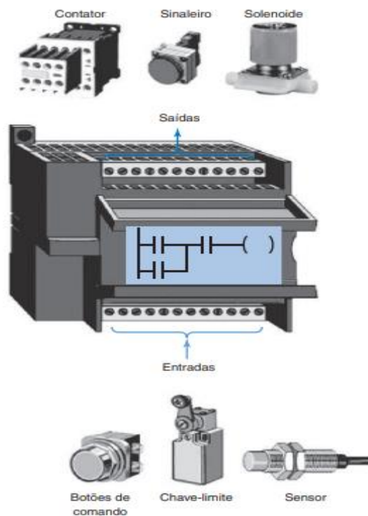
Figura 4: Entradas e saídas do CLP.
