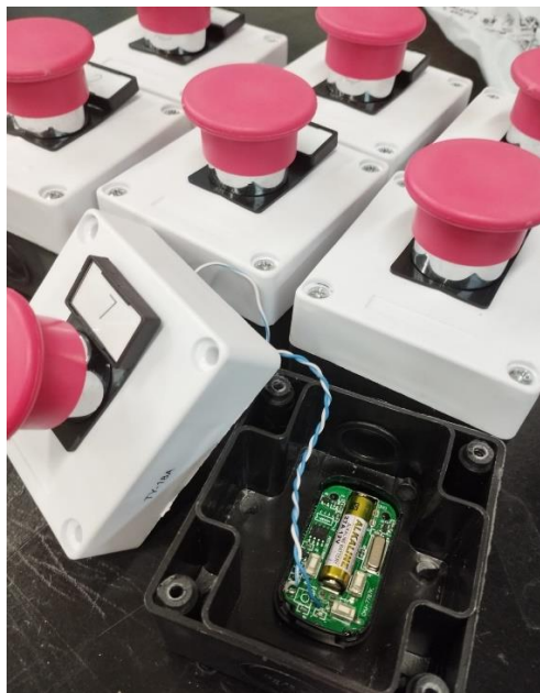
Figura 17 – Controle remoto.
